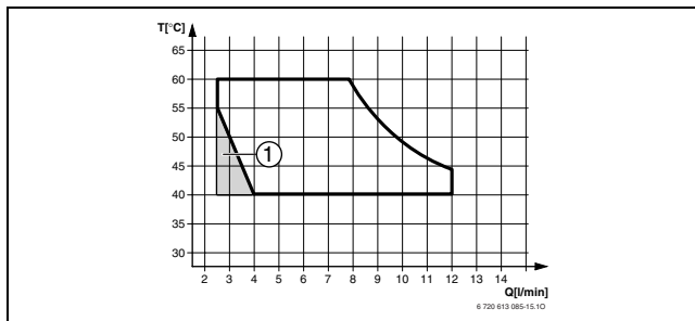
Рис 11 Диаграмма температуры подаваемой холодной воды от +15°C (ZWC 24)
